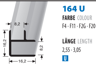
KOMBI INNEN- UND AUSSENECKE INTERIOR/EXTERIOR CORNER
