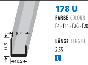
U-ABSCHLUSSPROFIL U BORDER PROFILE
