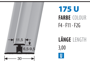
2-TEILIGER CLIP-VERBINDER 2-PART CLIP CONNECTOR
