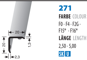
AUSSENWINKEL EXTERIOR ANGLE
