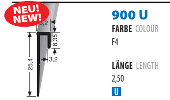
EINFASSPROFIL EDGE TRIM
