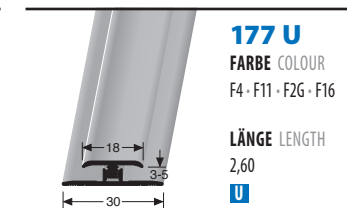
2-TEILIGER CLIP-VERBINDER 2-PART CLIP CONNECTOR
