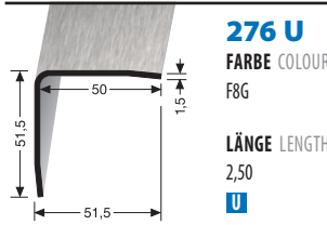
AUSSENWINKEL, 3-fach gekantet EXTERIOR ANGLE, 3-side edged
