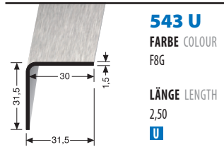
AUSSENWINKEL EXTERIOR ANGLE
